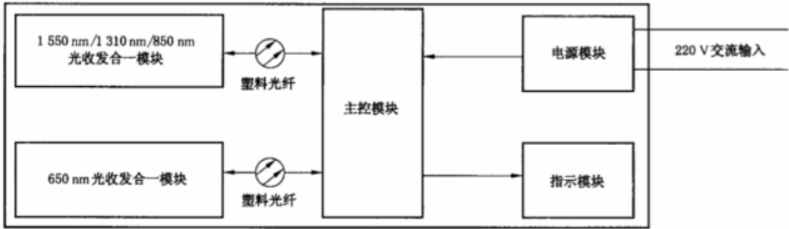
图 1 波长转换器的组成
