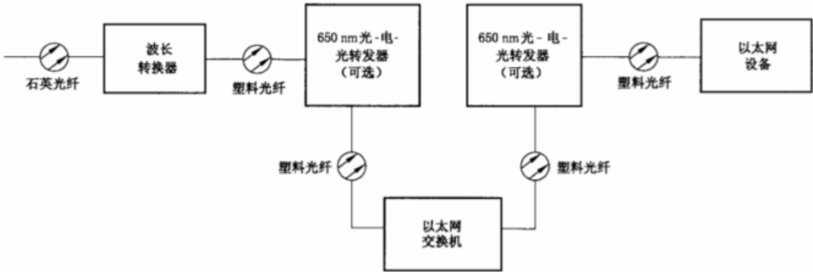
图 2 塑料光纤系统应用组成方框图
