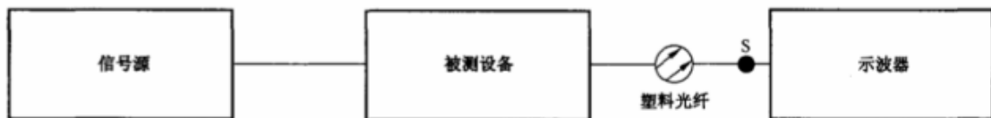
图 7 上升/下降时间测试配置
