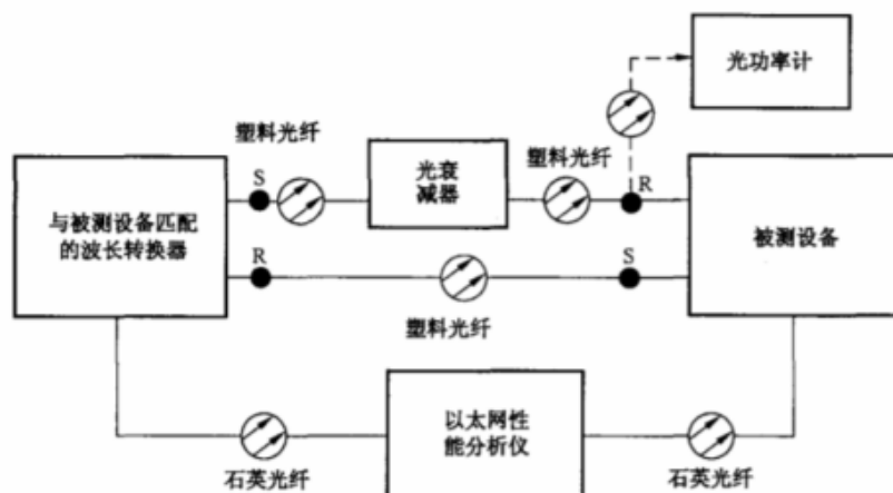
图 6 光接收灵敏度测试配置
